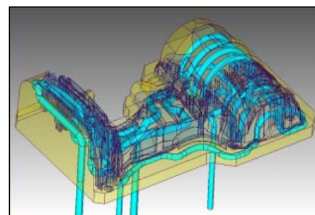
金型内部構造
