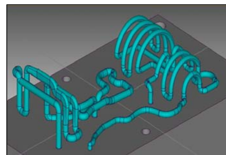
3次元連続水管の配置
