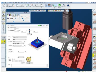
寸法計測 - 円内径
