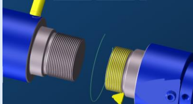
工具主軸とワーク主軸の 回転方向表示
