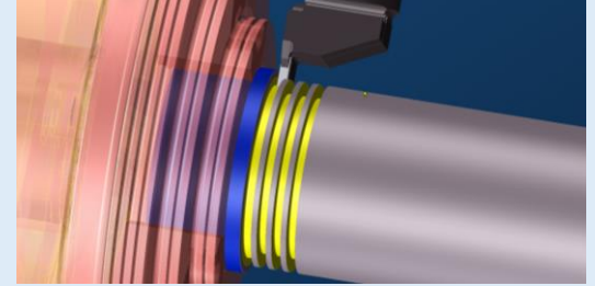
リブ切削プランジの加工シミュレーション
