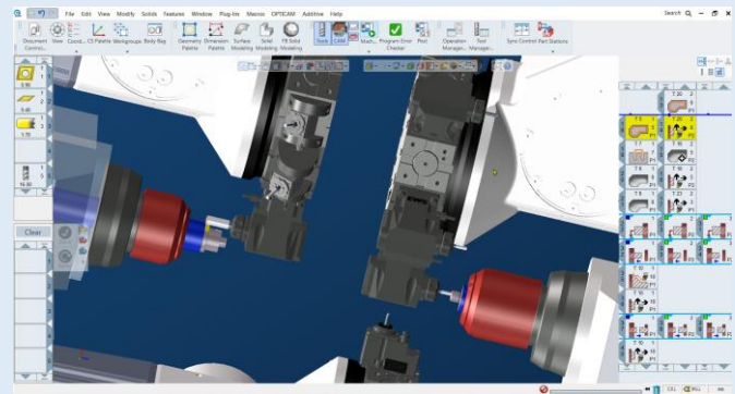
複合加工機(3ターレット)のマルチフロー並列表示 (同期フローモード)
