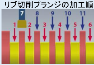
リブ切削プランジの加工シミュレーション
