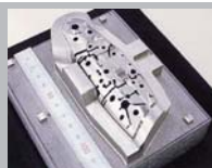
金属光造形複合加工機 LUMEX Avance-25
